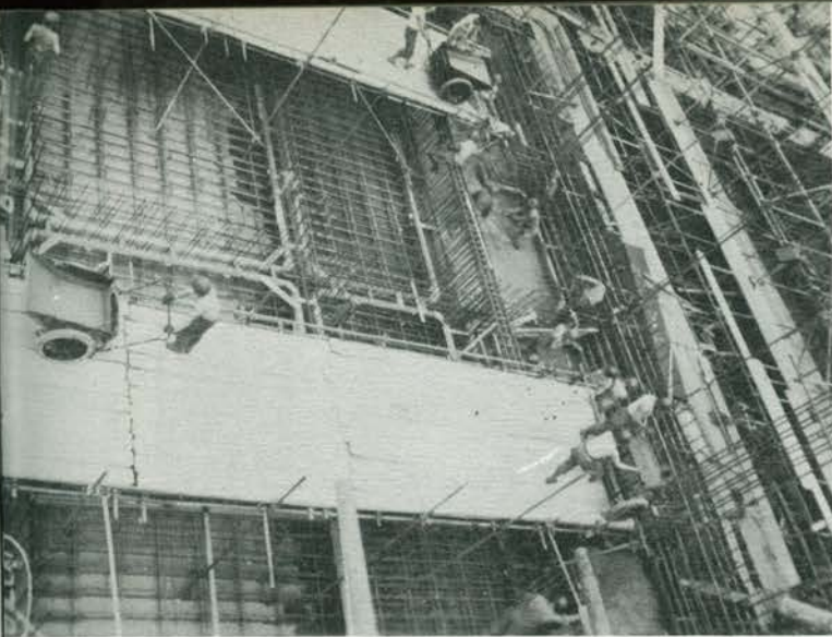
Pouring concrete
